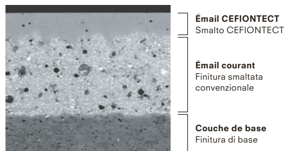
Micrographie WC CEFIONTECT * 1 \mu m=0,001 mm Micrografia di un vaso CEFIONTECT * 1 \mu m=0,001 mm
