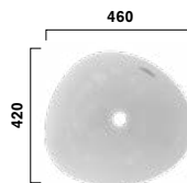
L4704E Aufsatzwaschtisch TA asymmetrisch 460mm, ohne Hahnloch, mit Überlauf Vessel TA, asymmetrical 460mm, without tap hole, with overflow
