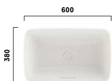
PJS06WEE#MW Aufsatzwaschtisch CE eckig, 600mm, ohne Hahnloch, mit Überlauf Vessel CE, square 600mm, without tap hole, with overflow
