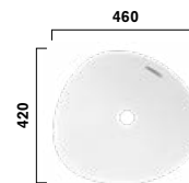
L4704E#MW Aufsatzwaschtisch TA asymmetrisch, matt Weiß, 460mm, ohne Hahnloch, mit Überlauf Vessel TA, asymmetrical, matte white, 460mm, without tap hole, with overflow
