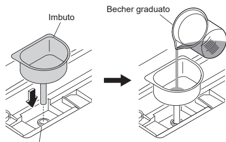
Porta disincrostazione
